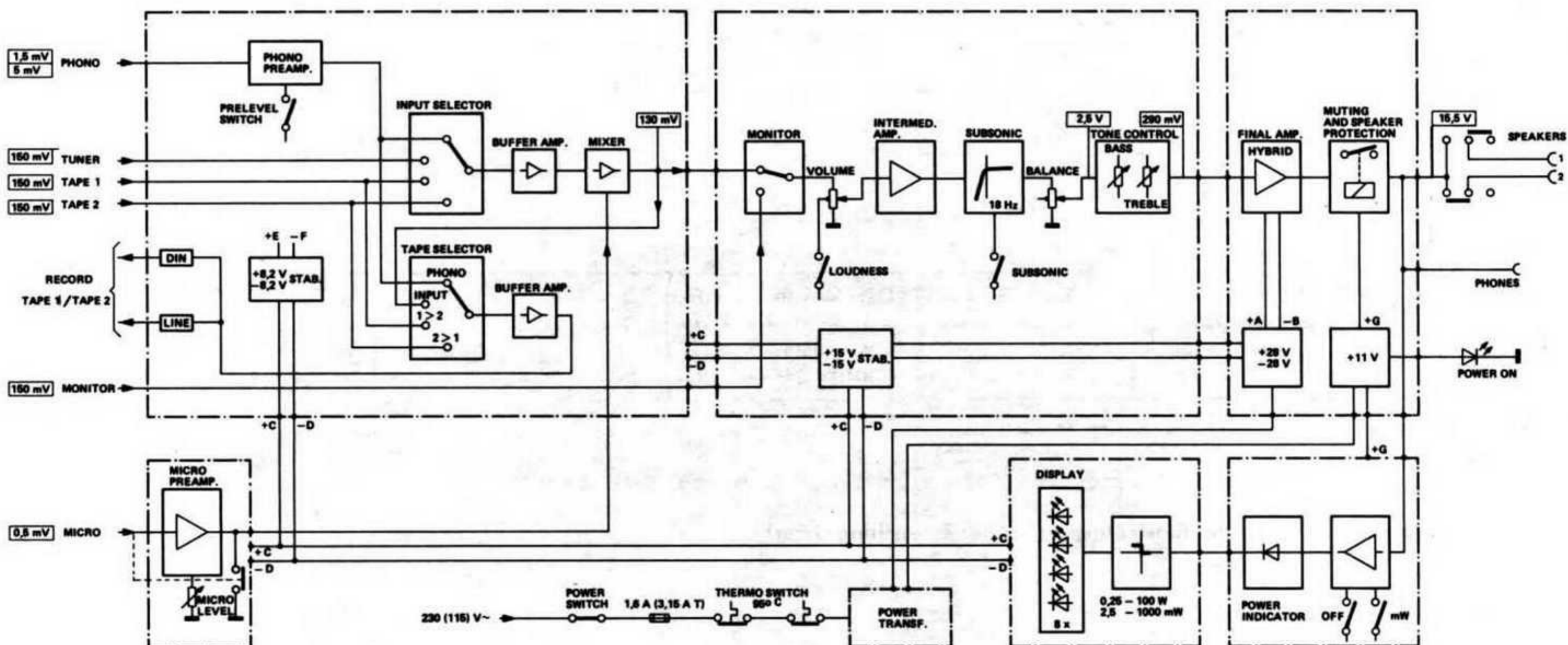
Blockschaltbild / Bloc diagram / Schéma de bloc
